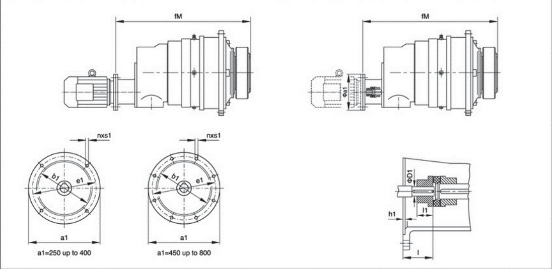
P3S. 带电机法兰及联轴器尺寸:
